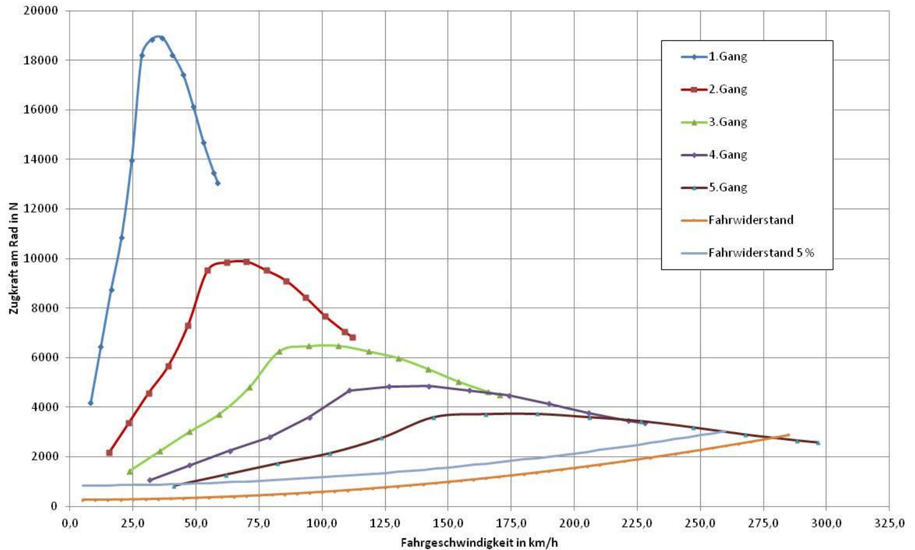
Zugkrafthyperbel C20LET Phase 3+ mit F18+ WR3,74
